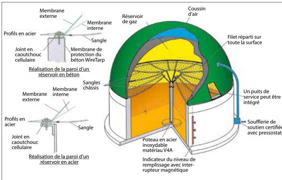
Réservoir à membrane double
